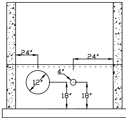
ELEVATION
